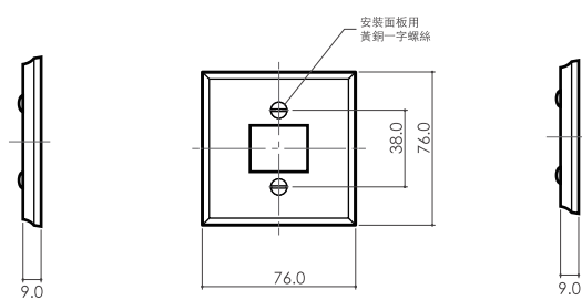
四角 一連一孔 代碼 CP-S-A
