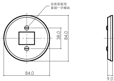
圓 一連一孔 代碼 CP-M-A
