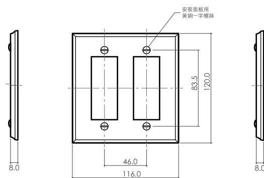
1112 二連四孔、六孔 代碼 CP-11-D
