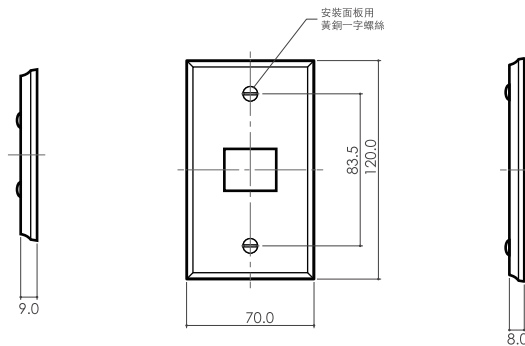
0712 一連一孔 代碼 CP-07-B
